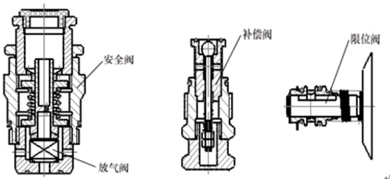
图3 放气安全阀
