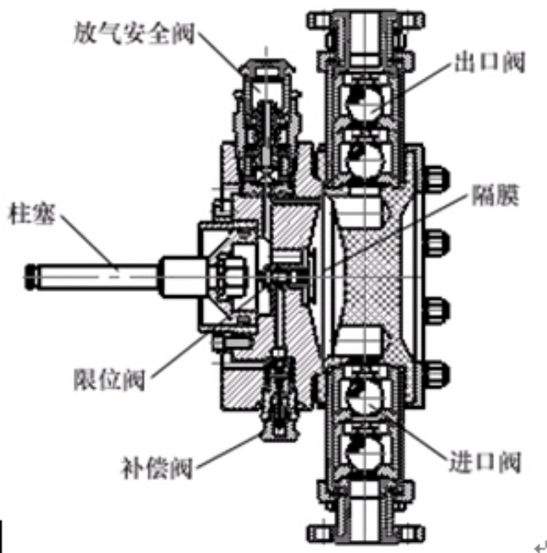
图2 隔膜式液力端结构示意图
