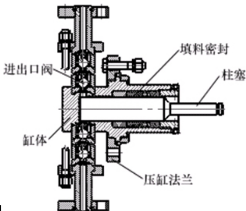
图1 柱塞式液力端结构示意图
